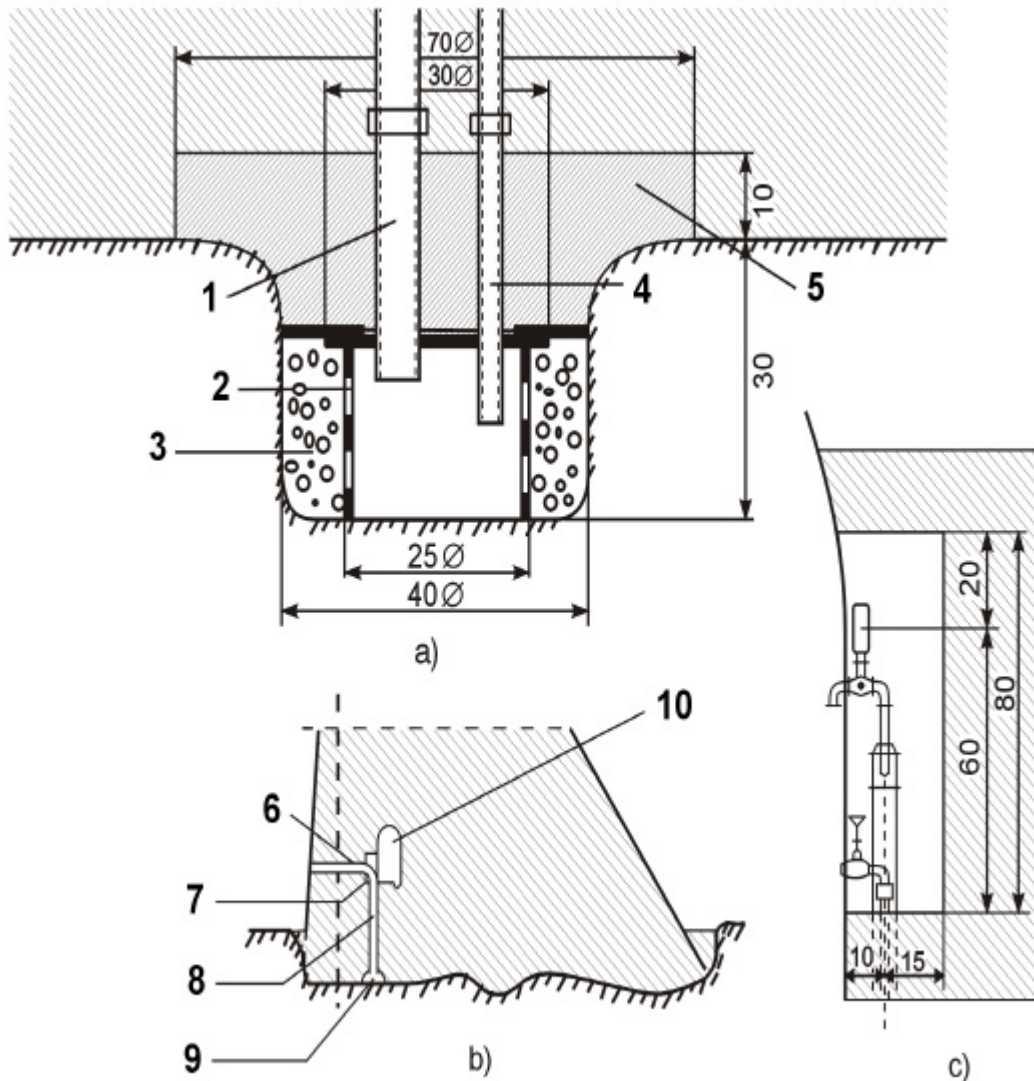
Fig 2 Mesures de sous-pression sous un mur-poids a) Récipient b) Technique de mesure dans le mur c) Niche d'armatures avec manomètre au tuyau de prise et conduite de rinçage (dessous) 1 Tuyau de prise 2 Récipient 3 Gravier filtrant 4 Tube de rinçage 5 Béton protecteur 6 Conduite de rinçage 7 Niche de mesure 8 Tuyau de prise 9 Récipient 10 Corridor
