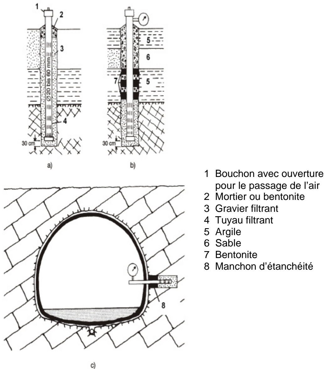
Fig 1 Figure schématique des mesures piézométriques.
